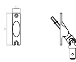
72 x 17mm - 45°
