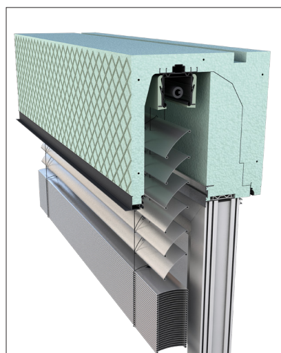
TERMOBOX-V
