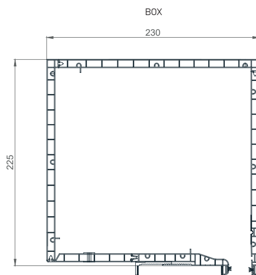
DIM. 230 X 225
