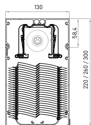
UNTERPUTZMONTAGE
