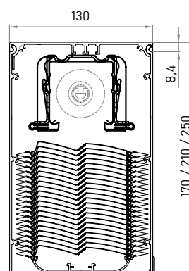
UNTERPUTZMONTAGE
