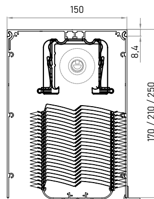
UNTERPUTZMONTAGE
