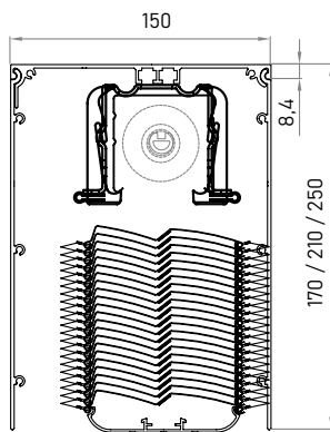
SICHTBARE MONTAGE
