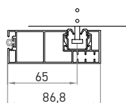
Führung KRATER 2G 31x87
