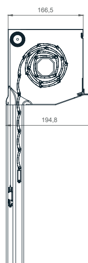
PODŽBUKNA 20° 165
