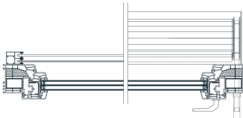
PODŽBUKNA 20° 137
