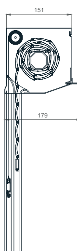
PODŽBUKNA 20° 150
