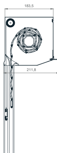
PODŽBUKNA 20° 180
