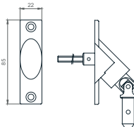
85 X 22mm - 90°
