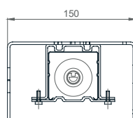
COMPACT (mogućnost ugradnje ROLO komarnika)
