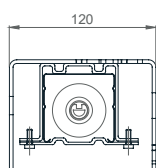
COMPACT (bez mogućnosti ugradnje ROLO komarnika)
