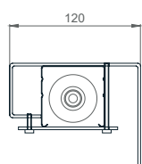
STANDARD (bez mogućnosti ugradnje ROLO komarnika)
