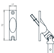
72 X 17mm - 45°
