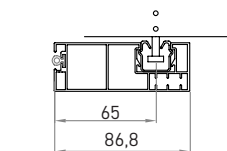
Führung KRATER 2G 31x87
