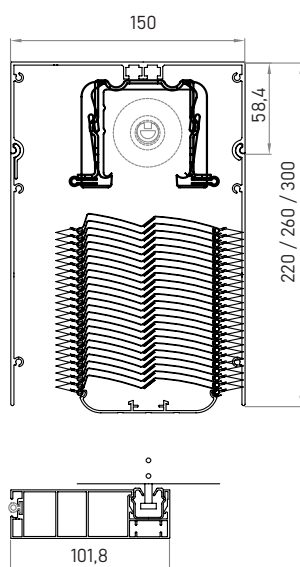
Führung KRATER 31x102
