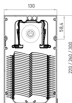
UNTERPUTZMONTAGE
