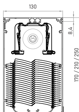
UNTERPUTZMONTAGE
