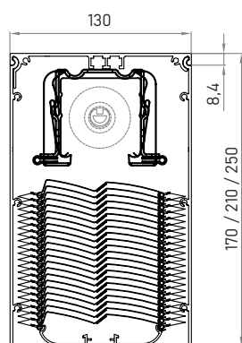
SICHTBARE MONTAGE
