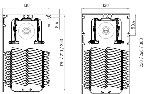
VIDNA VGRADNJA
