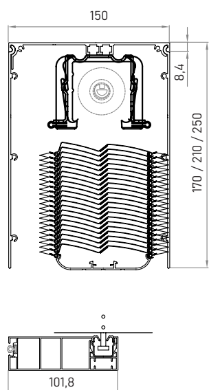
VIDNA VGRADNJA
