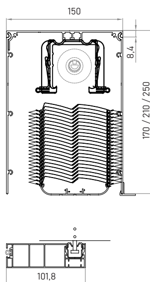
PODOMETNA VGRADNJA
