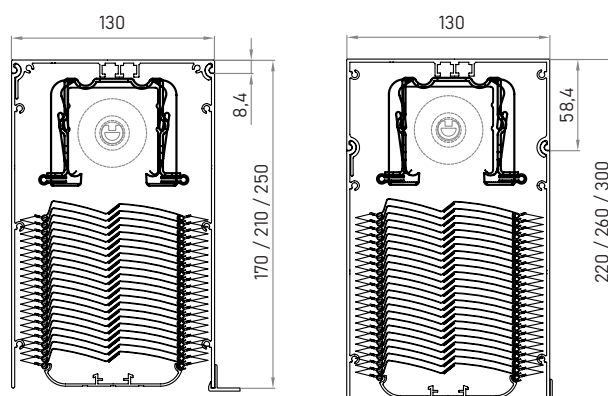
PODOMETNA VGRADNJA
