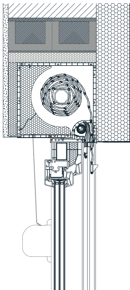
ZAMIK VODILA
