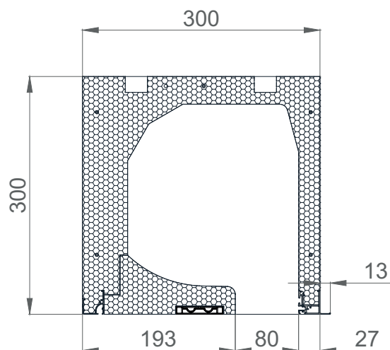
DIM. 300 X 300
